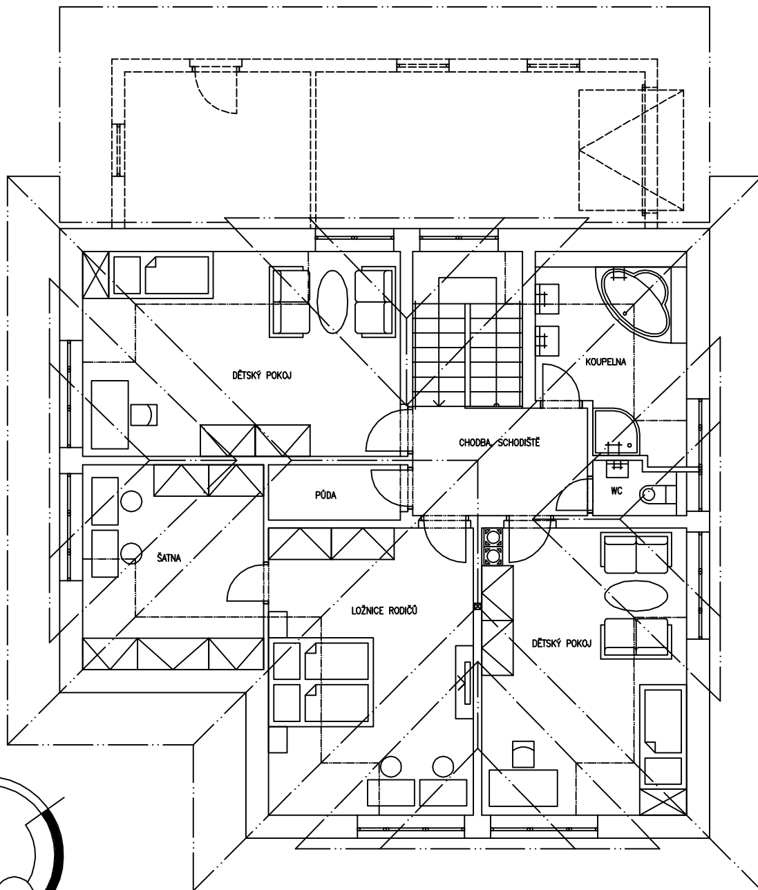
PODKROVÍ M 1:100
